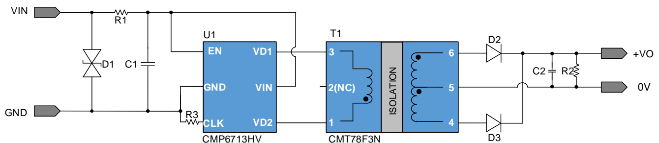
图 3.1 CMP6713HV 15V 输入, 5V 输出 2W 方案原理图
