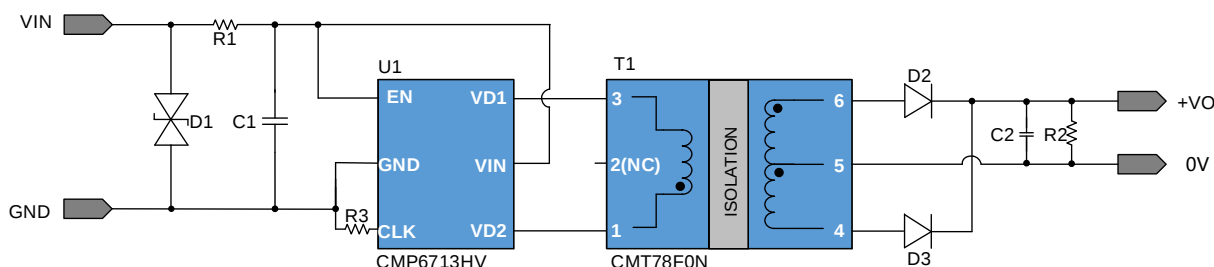
图 3.1 CMP6713HV 15V 输入, 15V 输出 2W 方案原理图
