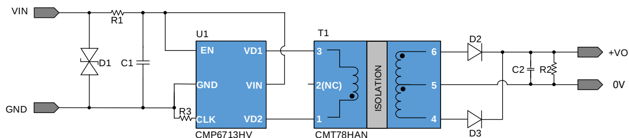
图 3.1 CMP6713HV 24V 输入, 5V 输出 2W 方案原理图
