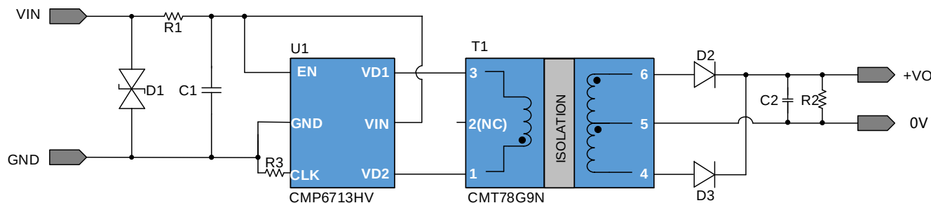
图 3.1 CMP6713HV 24V 输入, 9V 输出 2W 方案原理图
