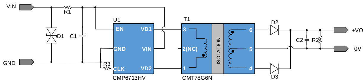
图 3.1 CMP6713HV 24V 输入, 15V 输出 2W 方案原理图
