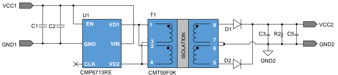
图 3.1 CMP6713RE 12V 输入, 12V 输出 2W 方案原理图
