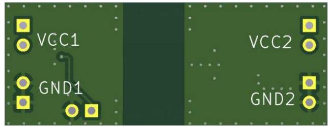
图 3.3 PCB 版图反面 (尺寸: 16 x 42mm)
