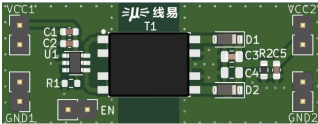
图 3.2 PCB 版图正面 (尺寸: 16 x 42mm)
