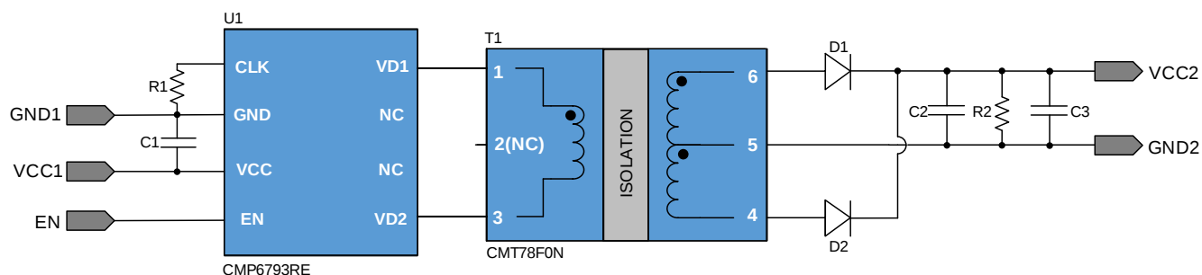
图 3.1 CMP6793RE 15V 输入, 15V 输出 3.5W 方案原理图
