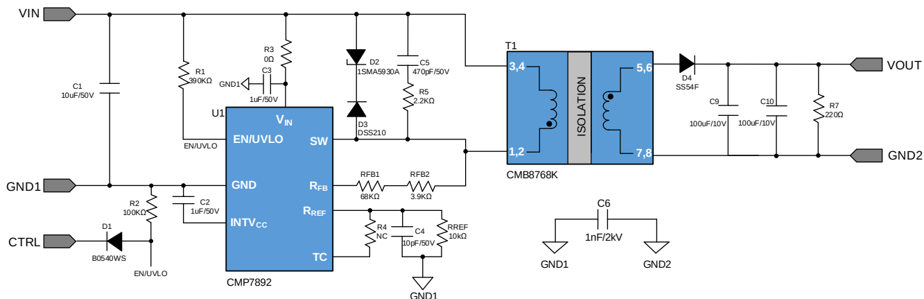
图 3.1 CMP7892 9-36V 输入 3.3V 输出 3W 方案原理图
