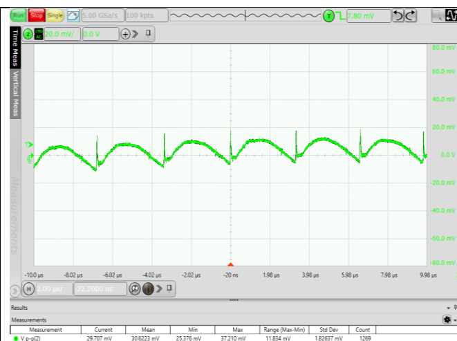
图 6.2 输出电压纹波波形 (VIN=24V, 100%负载)
