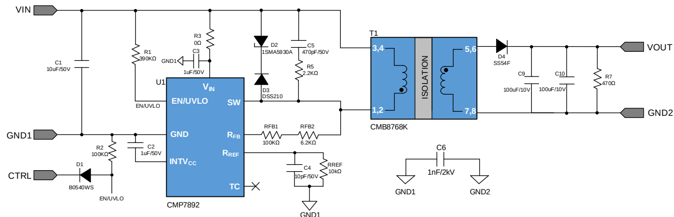
图 3.1 CMP7892 9-36V 输入 5V 输出 3W 方案原理图
