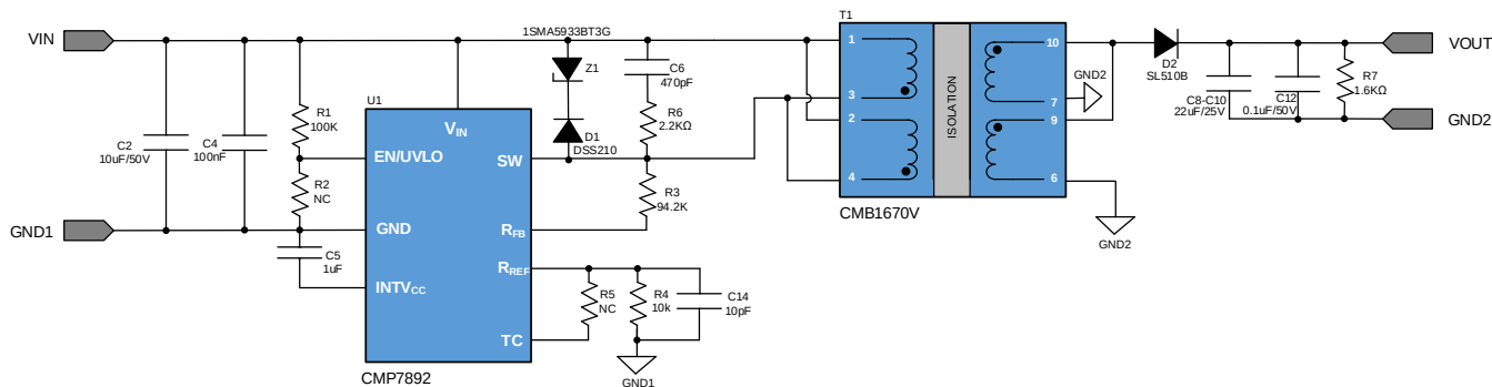
图 3.1 CMP7892 9-36V 输入 9V 输出 6W 方案原理图
