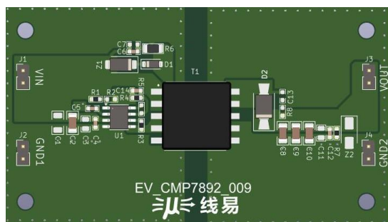
图 3.2 PCB 示意图 (尺寸: 45 x 80mm)
