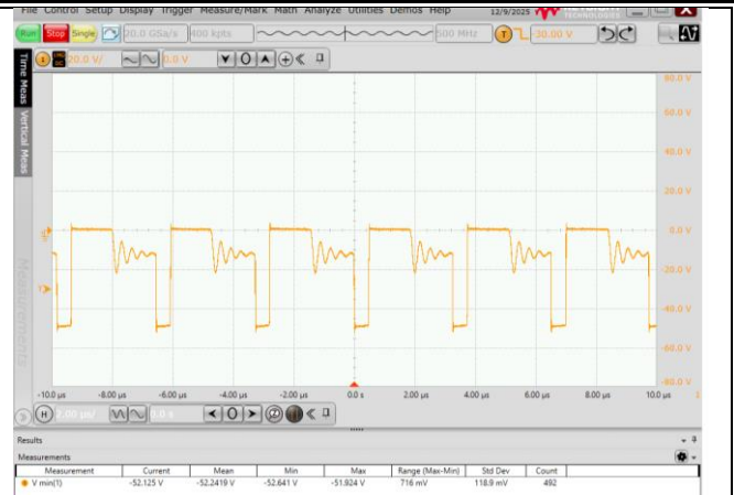
图 6.6 副边输出二极管应力波形 (VIN=36V, 满载)
