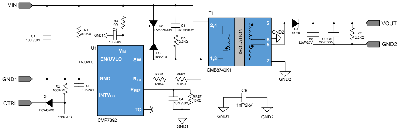
图 3.1 CMP7892 9-36V 输入 12V 输出 3W 方案原理图
