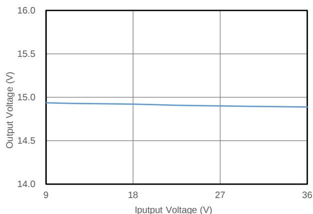
图 5.3 输出电压 vs 输入电压 (满载)
