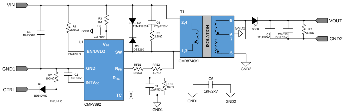
图 3.1 CMP7892 9-36V 输入 15V 输出 3W 方案原理图
