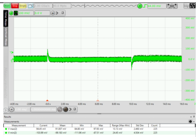
图 6.4 50% -75% -50%IO 动态波形 (VIN=24V)
