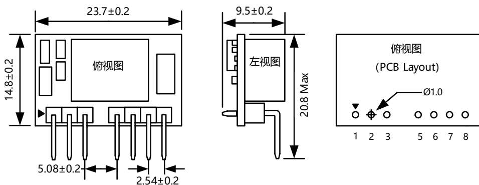
图 3.2 方案外形图
