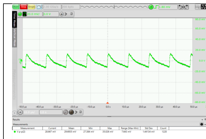
图 6.1 输出电压纹波波形 (VIN=24V, 5%负载)
