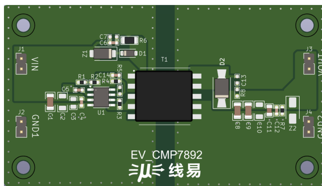
图 3.2 PCB 示意图 (尺寸: 45 x 80mm)
