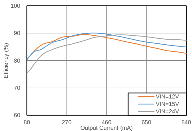
图 5.1 输出电压 vs 输出电流 (常温)
