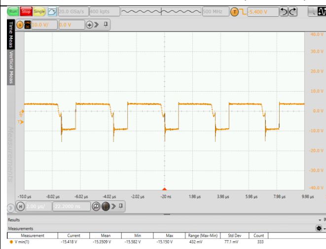
图 6.4 50% -75% -50%IO 动态波形 (VIN=12V)
