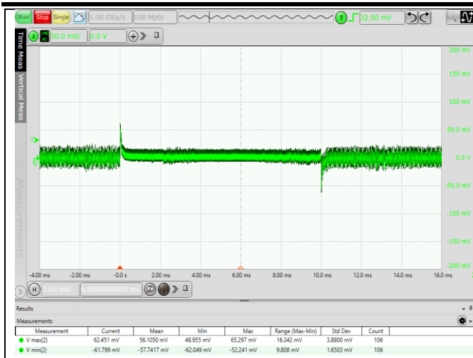
图 6.3 25% -50% -25%IO 动态波形 (VIN=12V)
