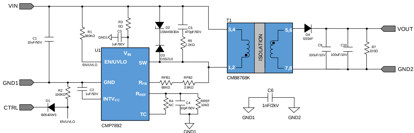
图 3.1 CMP7892 9-18V 输入 3.3V 输出 3W 方案原理图
