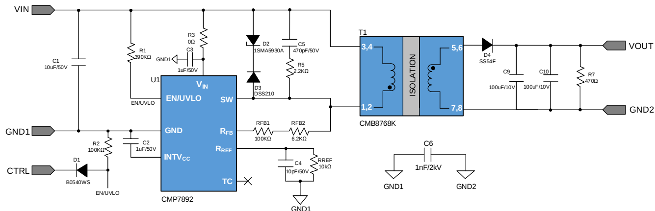
图 3.1 CMP7892 9-18V 输入 5V 输出 3W 方案原理图
