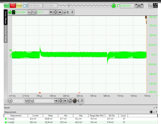
图 6.4 50% -75% -50%IO 动态波形 (VIN=12V)
