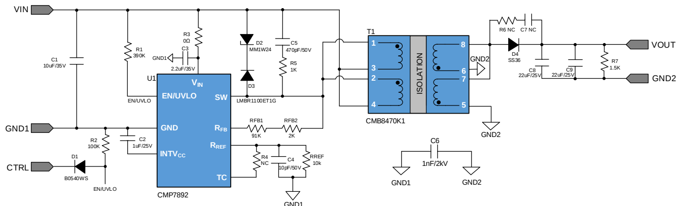
图 3.1 CMP7892 9-18V 输入 9V 输出 3W 方案原理图
