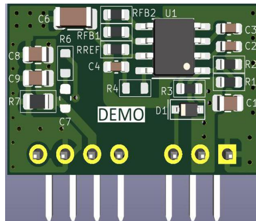
图 3.4 PCB 版图反面
