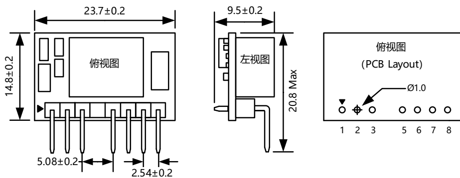
图 3.2 方案外形图
