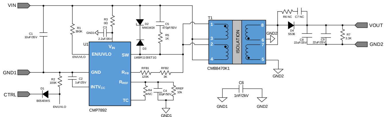
图 3.1 CMP7892 9-18V 输入 12V 输出 3W 方案原理图
