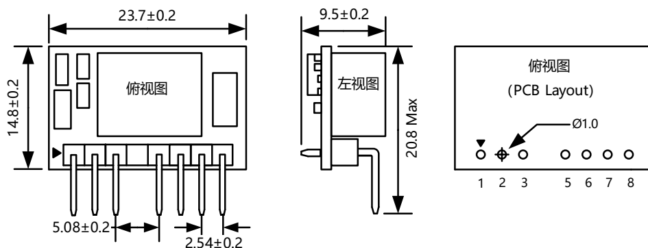
图 3.2 方案外形图
