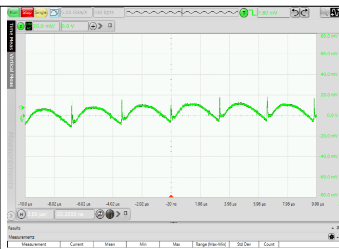
图 6.2 输出电压纹波波形 (VIN=24V, 100%负载)
