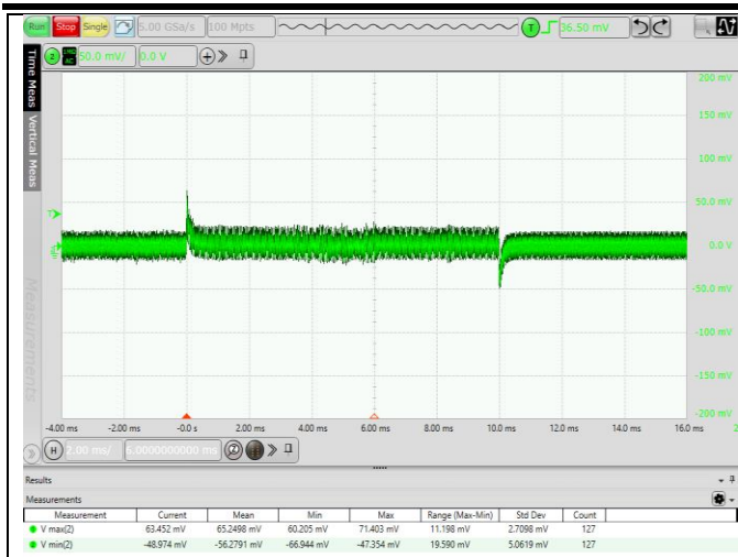
图 6.3 25% -50% -25%IO 动态波形 (VIN=24V)
