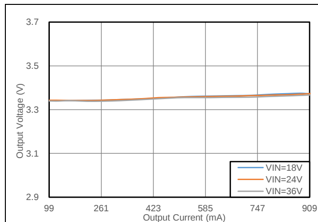
图 5.1 输出电压 vs 输出电流
