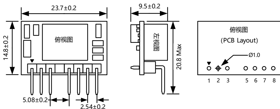
图 3.2 方案外形图
