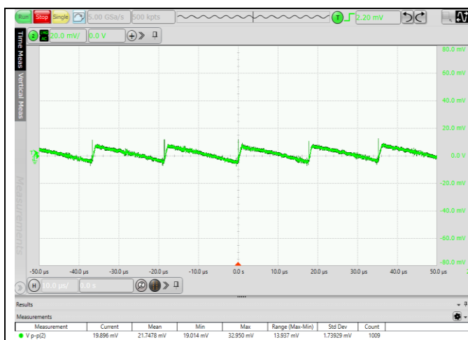
图 6.1 输出电压纹波波形 (VIN=24V, 5%负载)
