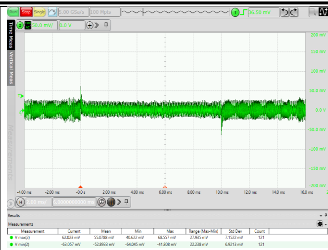
图 6.4 50% -75% -50%IO 动态波形 (VIN=24V)
