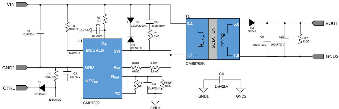
图 3.1 CMP7892 18-36V 输入 3.3V 输出 3W 方案原理图
