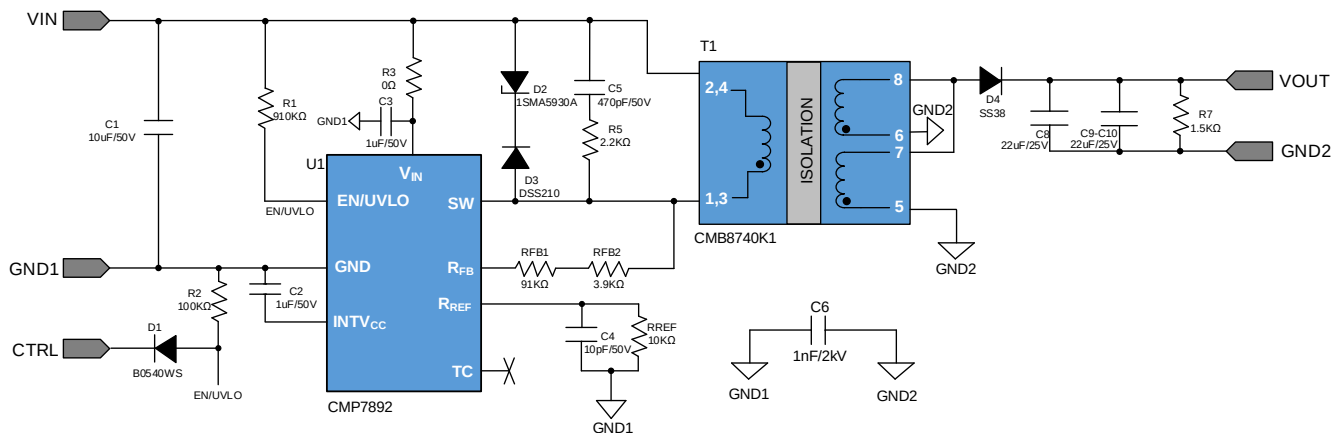
图 3.1 CMP7892 18-36V 输入 9V 输出 3W 方案原理图
