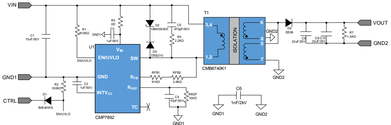
图 3.1 CMP7892 18-36V 输入 9V 输出 3W 方案原理图
