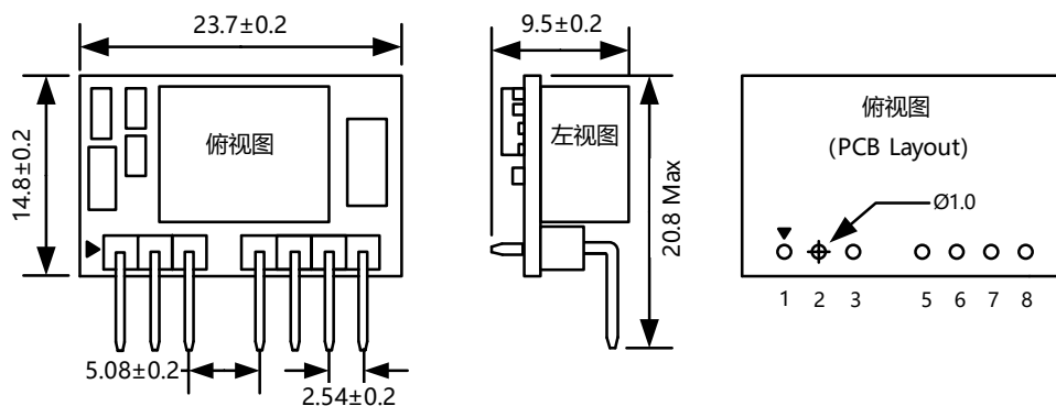
图 3.2 方案外形图
