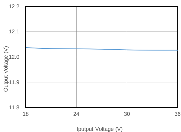
图 5.3 输出电压 vs 输入电压 (满载)
