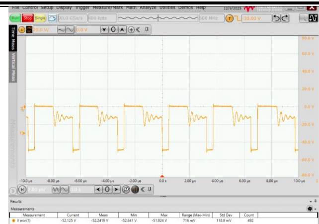
图 6.6 副边输出二极管应力波形 (VIN=36V, 满载)
