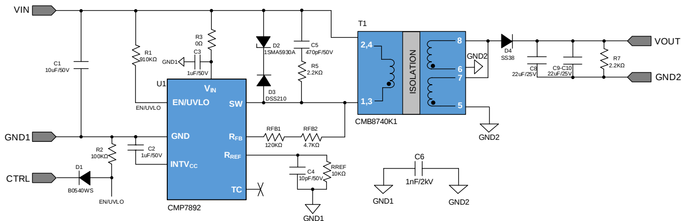
图 3.1 CMP7892 18-36V 输入 12V 输出 3W 方案原理图
