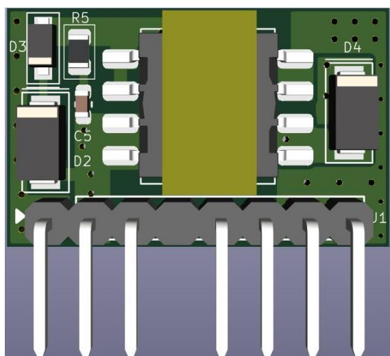
图 3.3 PCB 版图正面
