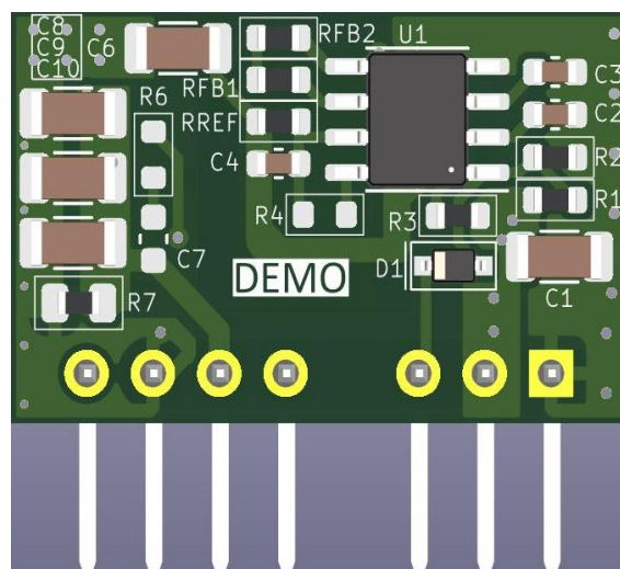
图 3.4 PCB 版图反面
