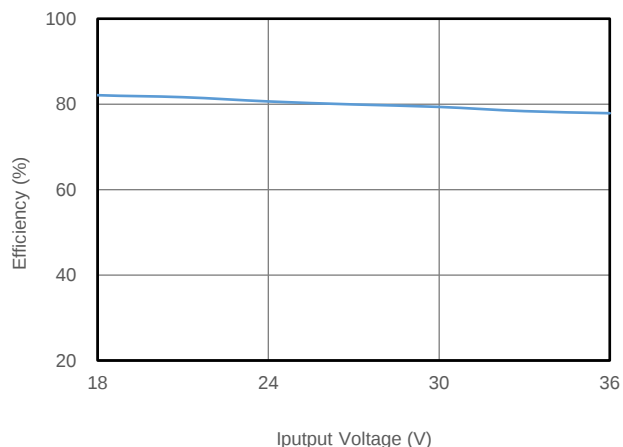
图 5.4 转换效率 vs 输入电压 (满载)
