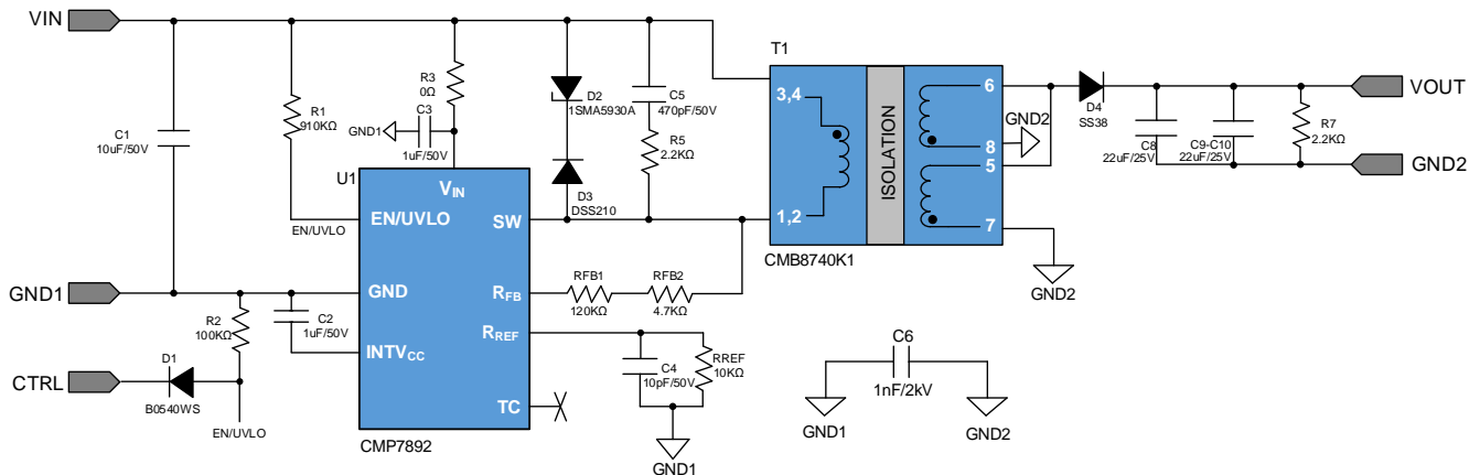
图 3.1 CMP7892 18-36V 输入 12V 输出 3W 方案原理图
