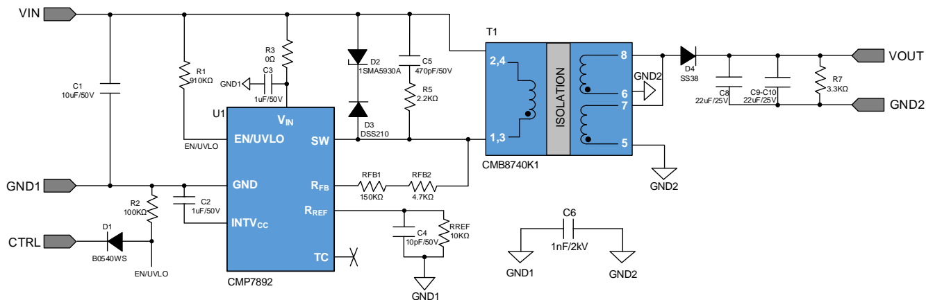
图 3.1 CMP7892 18-36V 输入 15V 输出 3W 方案原理图
