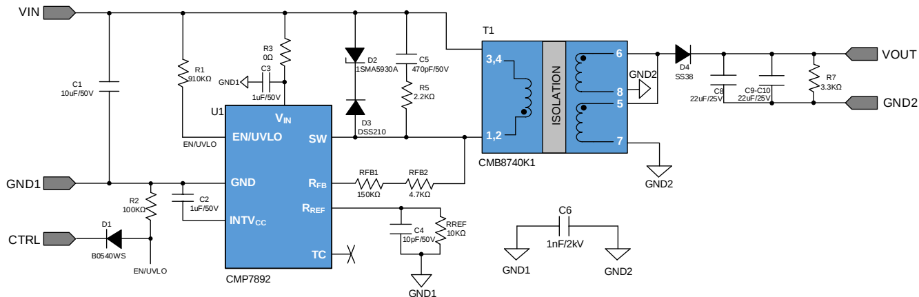
图 3.1 CMP7892 18-36V 输入 15V 输出 3W 方案原理图
