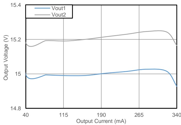
图 5.9 输出电压 vs 输出电流 ( V_{IN}=36V )
