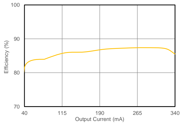
图 5.8 转换效率 vs 输出电流 ( V_{IN}=24V )
