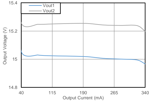
图 5.5 输出电压 vs 输出电流 ( V_{IN}=15V )
