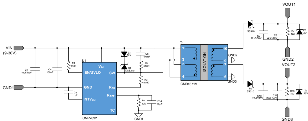
图 3.1 CMP7892 9-36V 输入双路 15V 和 15V 输出 10W 方案原理图
