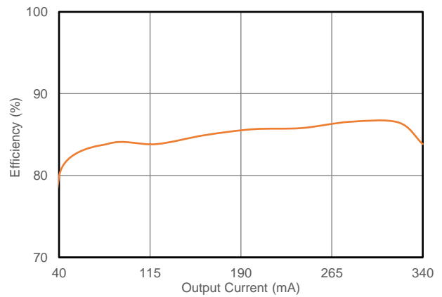
图 5.10 转换效率 vs 输出电流 ( V_{IN}=36V )
