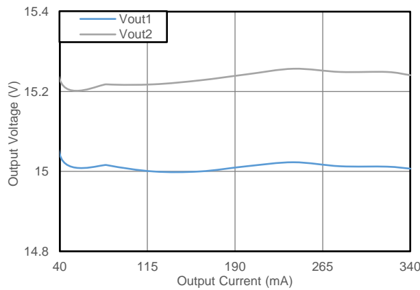
图 5.7 输出电压 vs 输出电流 ( V_{IN}=24V )
