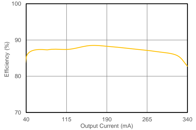
图 5.6 转换效率 vs 输出电流 ( V_{IN}=15V )
